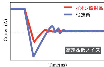
ダイオードのリカバリー波形比較イメージ
