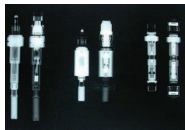
左: X線撮影 右: 中性子撮影
