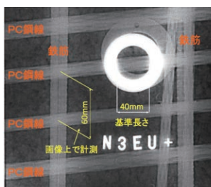
PC桁内部検査
